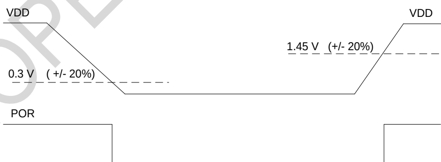
图 4. 电源电压下降导致 POR 复位
