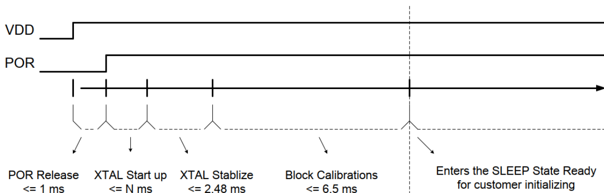
图 12.上电时序
