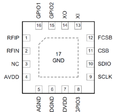
CMT2219B 顶视图
