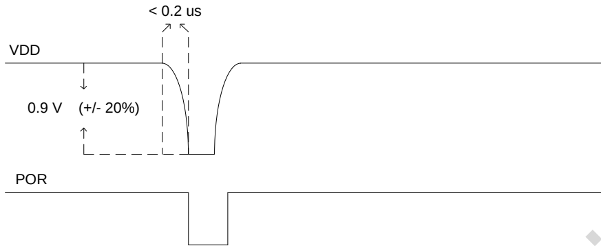
图 5. 电源电压迅速下降导致 POR 复位
