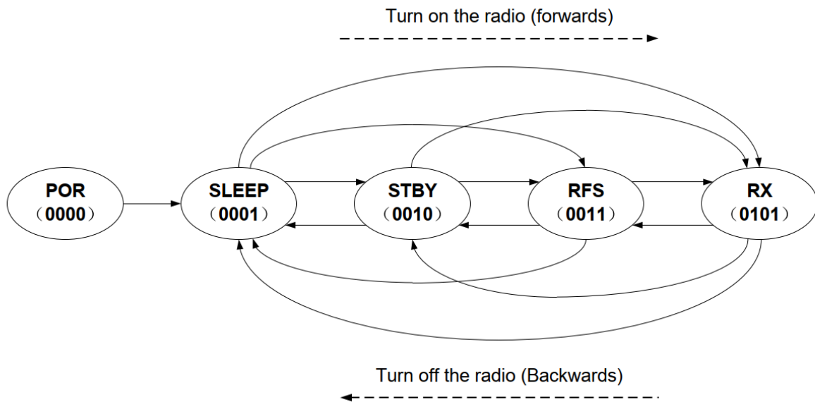
图 13.状态切换图
